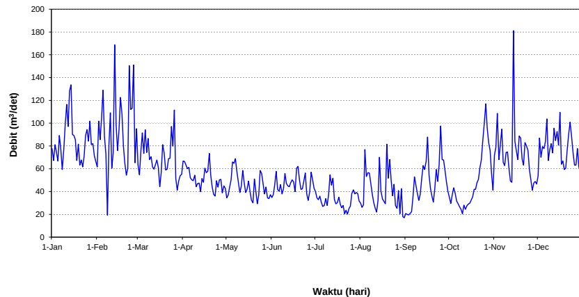
HIDROGRAF DEBIT HARIAN (m 3 /dt) S.KLawing-SLInga TAHUN 2022
