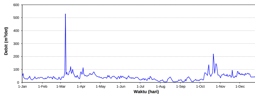
HIDROGRAF DEBIT HARIAN (m 3 /dt) S.SERAYU-BANJARNEGARA TAHUN 2022
