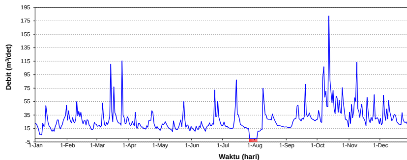
HIDROGRAF DEBIT HARIAN (m 3 /dt) S.TAJUM-TIPARKIDUL TAHUN 2022
