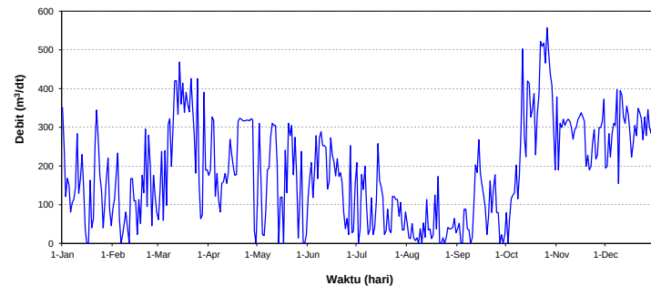
HIDROGRAF DEBIT HARIAN (m 3 /dt) S.SERAYU-GUMIWANG TAHUN 2022
