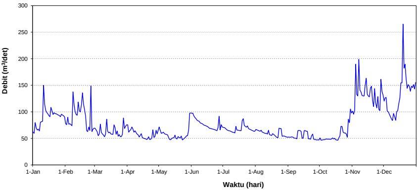
HIDROGRAF DEBIT HARIAN (m³/dt) S.MERAWU-CLANGAP TAHUN 2022
