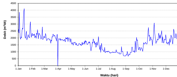
HIDROGRAF DEBIT HARIAN (m 3 /dt) S.SERAYU-RAWALO TAHUN 2021
