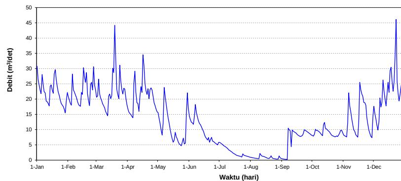
HIDROGRAF DEBIT HARIAN (m 3 /dt) S.BEGALUH -KRASAK TAHUN 2022
