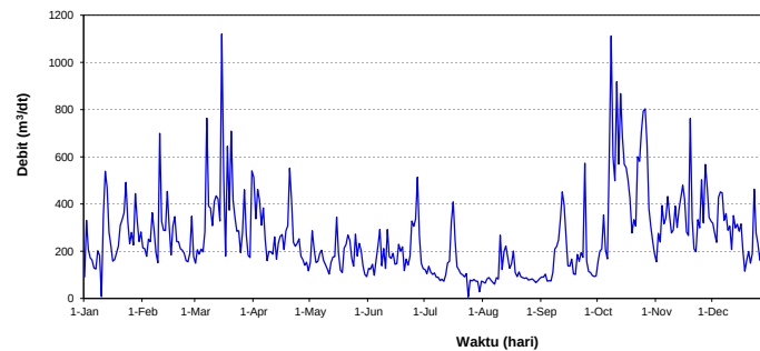
HIDROGRAF DEBIT HARIAN (m 3 /dt) S.SERAYU-BANYUMAS TAHUN 2022
